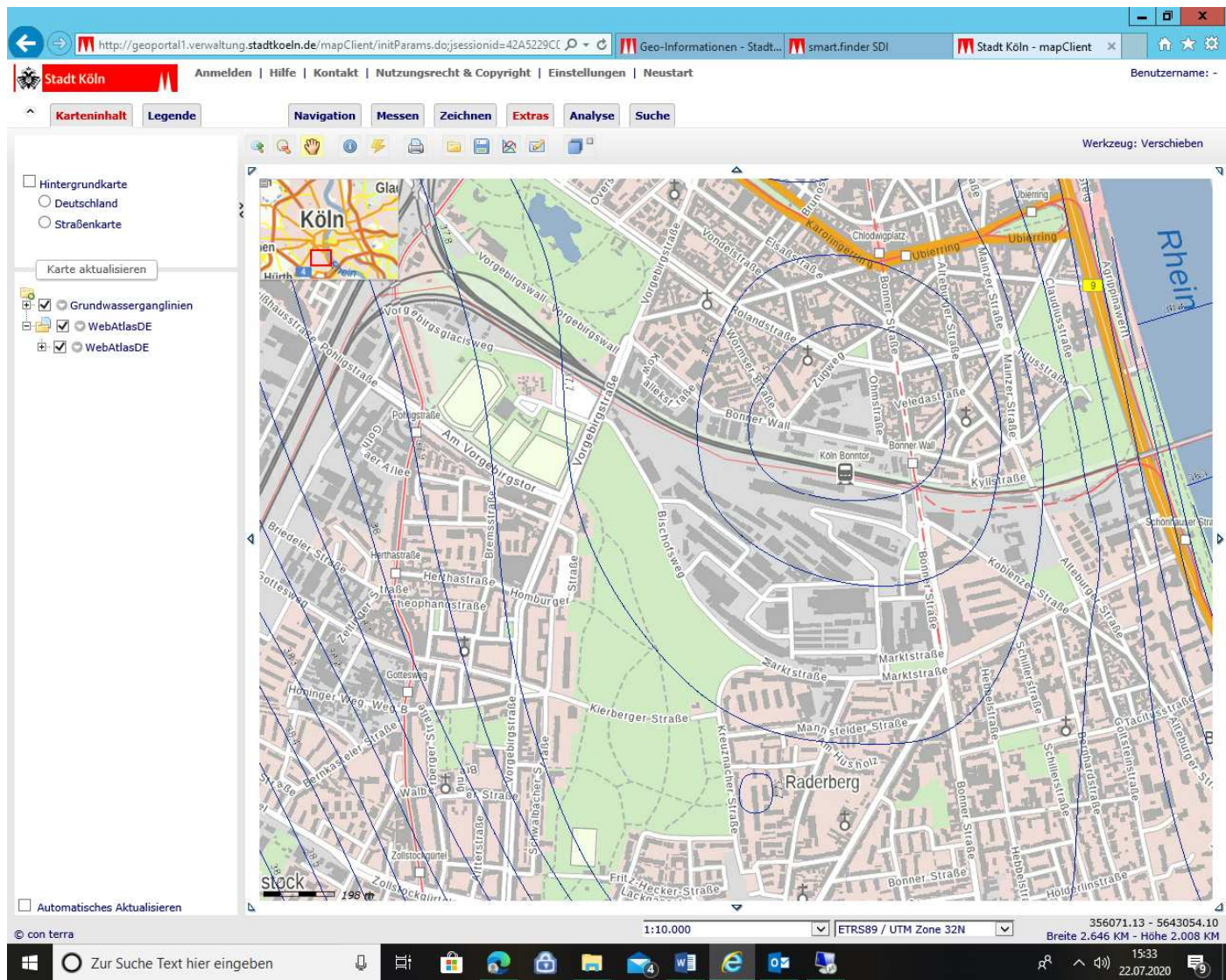
Mittlere Grundwassergleichen 10/2003 (GEW)
