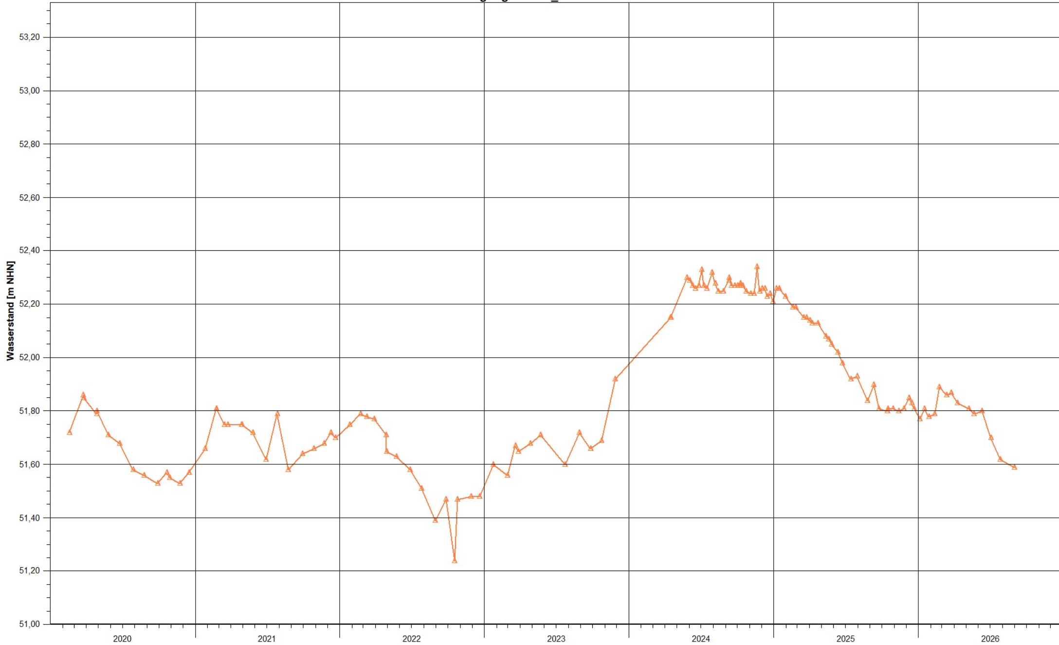
Grundwasserganglinie RS_47 01.01.2020 - 31.08.2026
