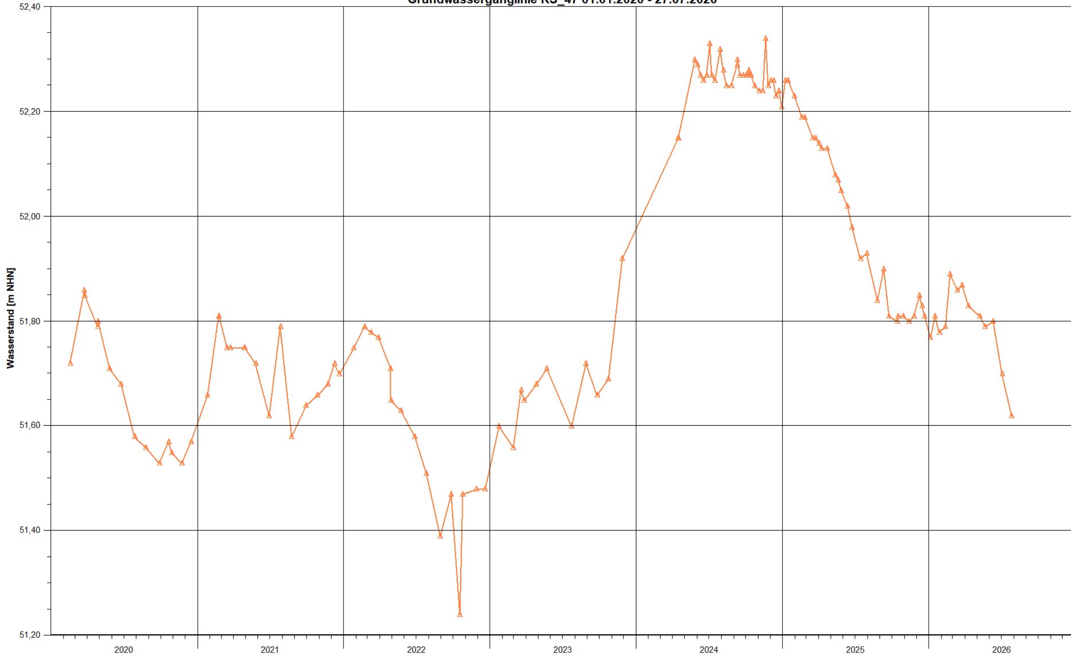
Grundwasserganglinie RS_47 01.01.2020 - 27.07.2026
