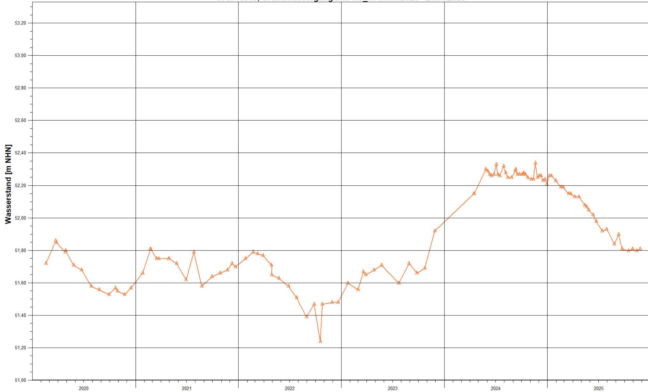
076748315, Grundwasserganglinie RS_47 01.01.2020 - 25.11.2025
