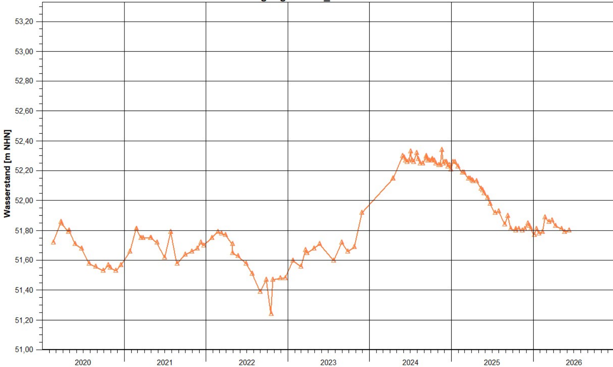
Grundwasserganglinie RS_47 01.01.2020 - 11.06.2026
