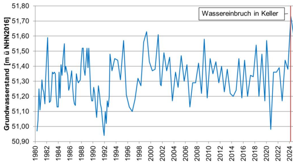
Abb. 7: Ganglinie der GWM 076917812 östlich des hydr. Sprungs, Wohngebiet Lind
