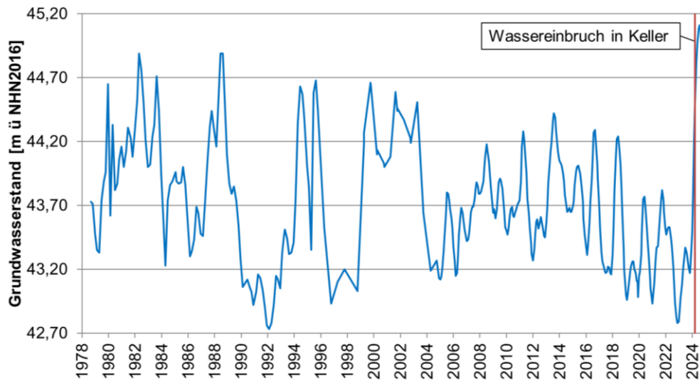
Abb. 1: Ganglinie der GWM 076704610 westlich des hydr. Sprungs, Gewerbegebiet Lind
