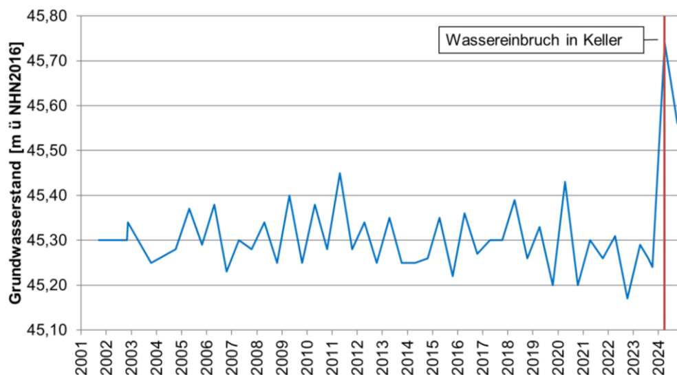
Abb. 10: Ganglinie der GWM 076943215 westlich des hydr. Sprungs, entlang Rheinkanal I
