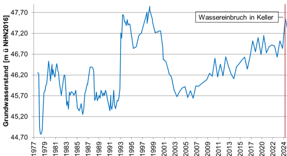
Abb. 3: Ganglinie der GWM 076704117 westlich des hydr. Sprungs, Gewerbegebiet Lind
