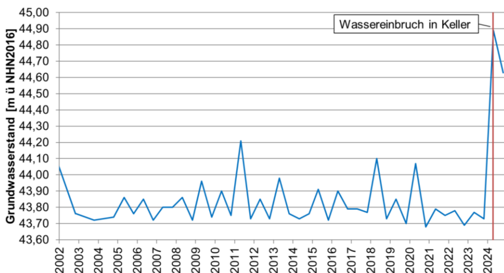
Abb. 11: Ganglinie der GWM 076943318 westlich des hydr. Sprungs, entlang Rheinkanal I
