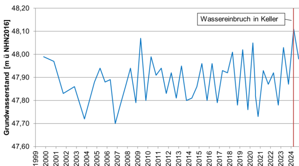
Abb. 12: Ganglinie der GWM 076943410 östlich des hydr. Sprungs, entlang Rheinkanal I
