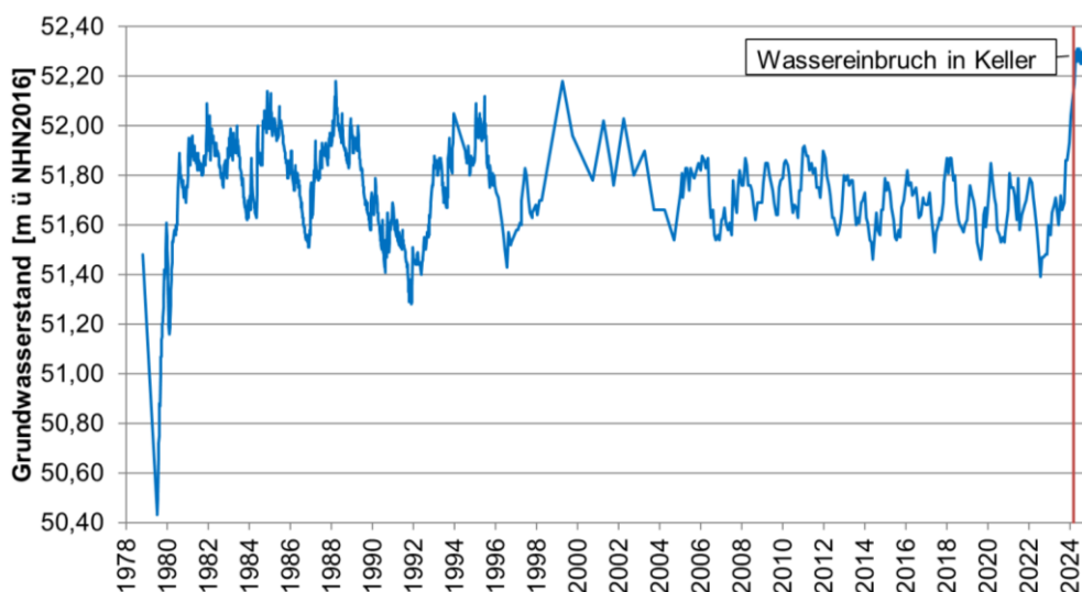
Abb. 6: Ganglinie der GWM 076748315 östlich des hydr. Sprungs, Schilfweg
