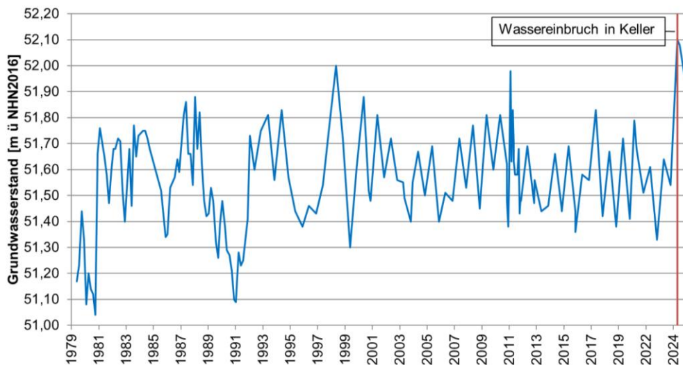
Abb. 5: Ganglinie der GWM 076917915 östlich des hydr. Sprungs, Schilfweg
