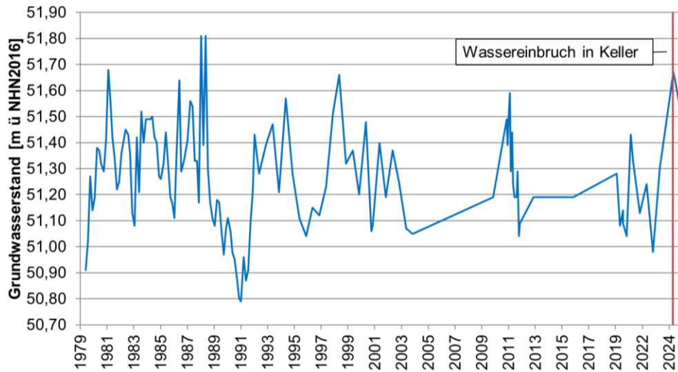
Abb. 4: Ganglinie der GWM 076918117 östlich des hydr. Sprungs, Schilfweg
