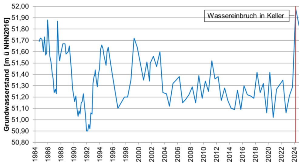
Abb. 8: Ganglinie der GWM 076918518 östlich des hydr. Sprungs, Wohngebiet Lind
