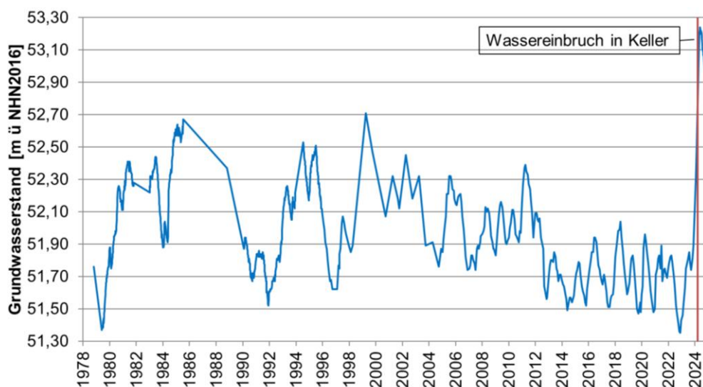
Abb. 9: Ganglinie der GWM 076748418 östlich des hydr. Sprungs, Wohngebiet Lind
