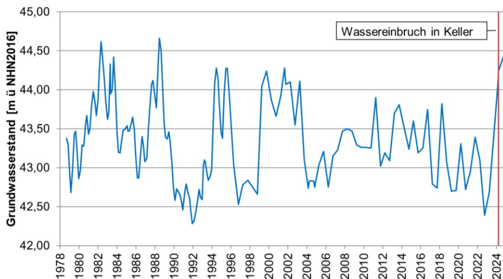
Abb. 2: Ganglinie der GWM 076704415 westlich des hydr. Sprungs, Gewerbegebiet Lind
