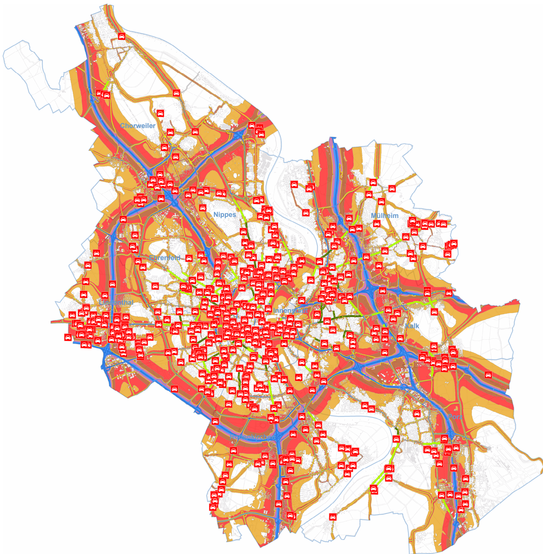
Vorschläge Straßenlärm - Mittelungspegel 24 h (Lden) - Belastungsschwerpunkte
