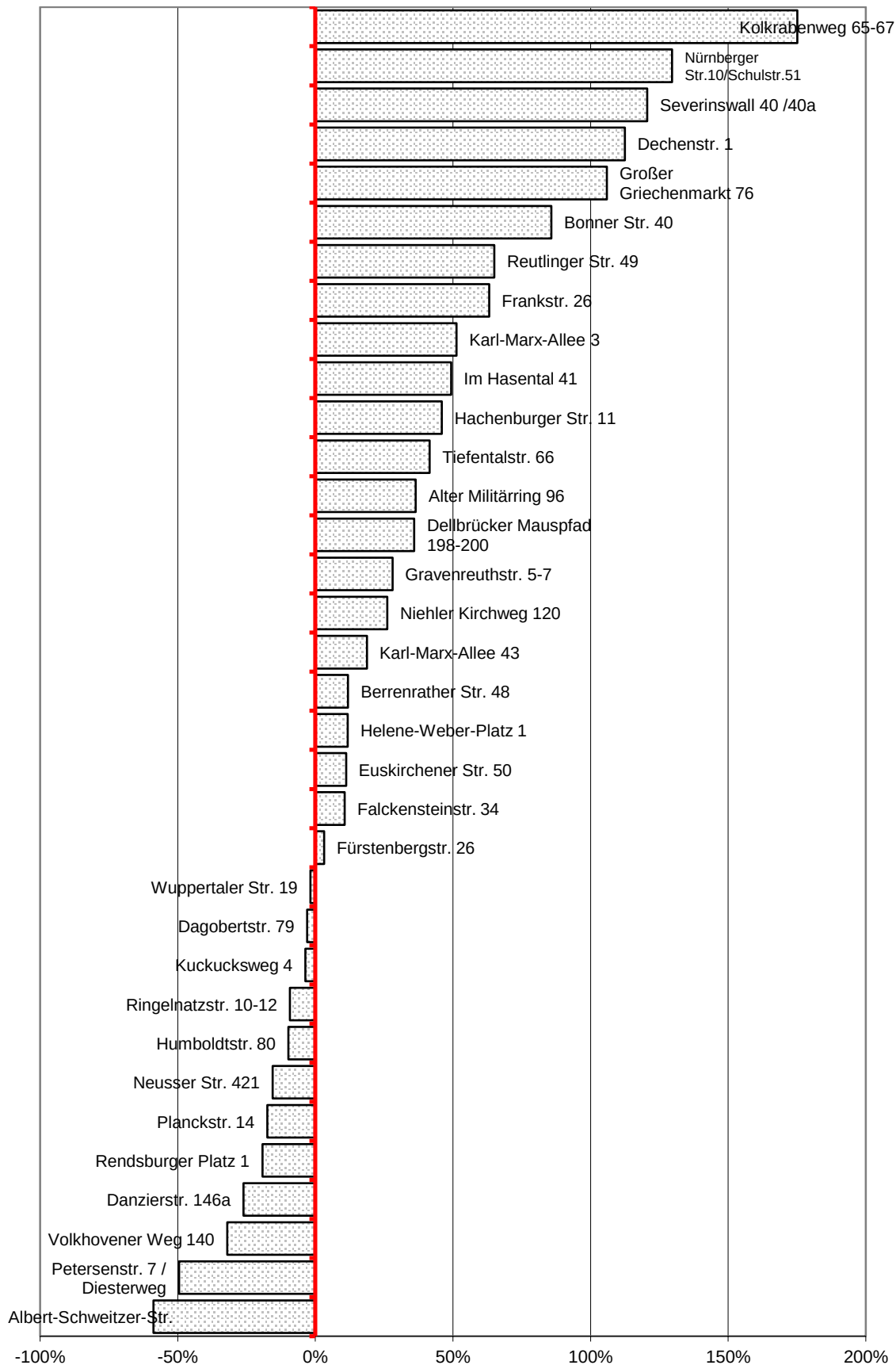
Abbildung A2.9: Haupt- und Realschulen, Heizung
