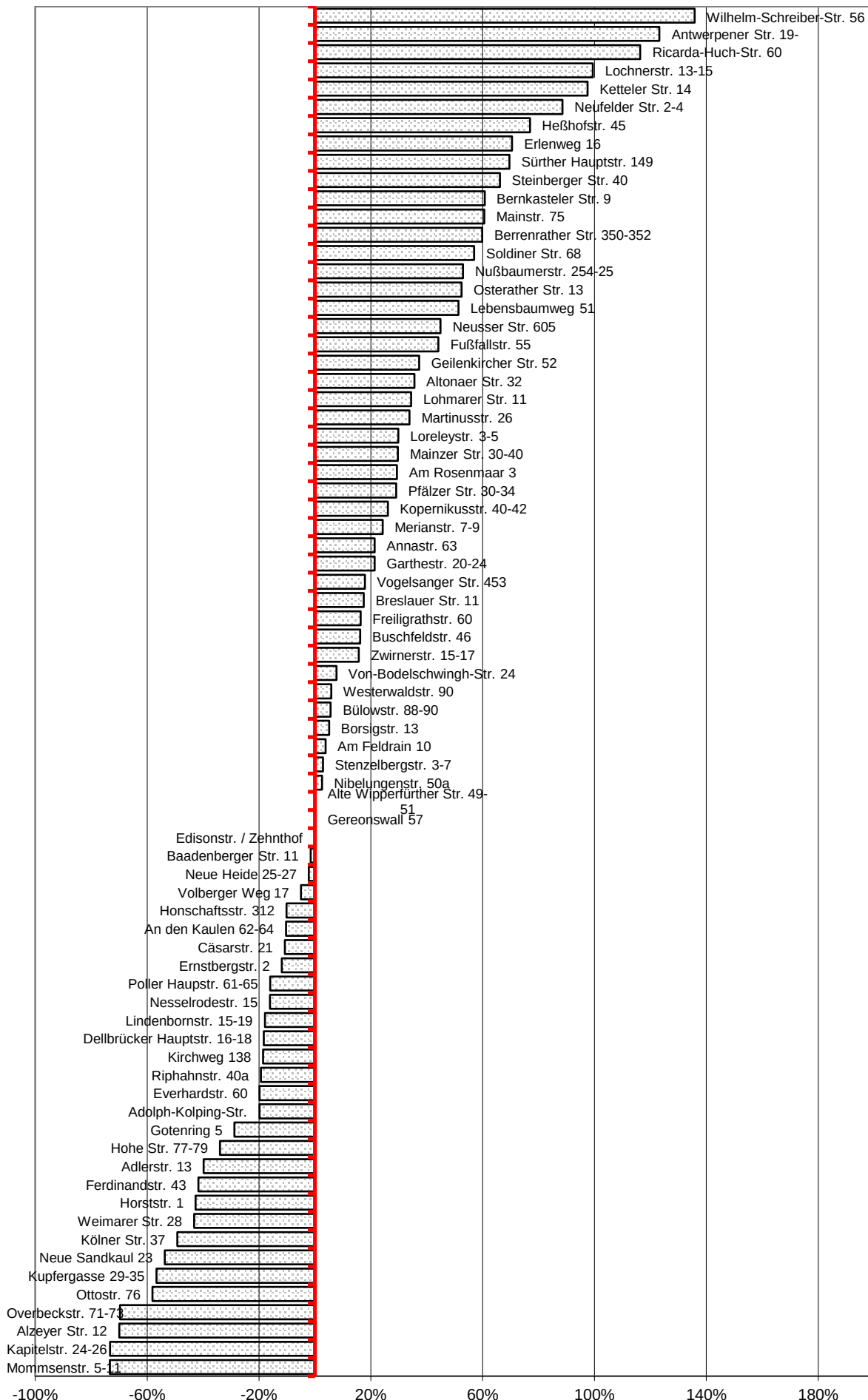
Abbildung A2.3: Grundschulen > 3.500 m², Heizung
