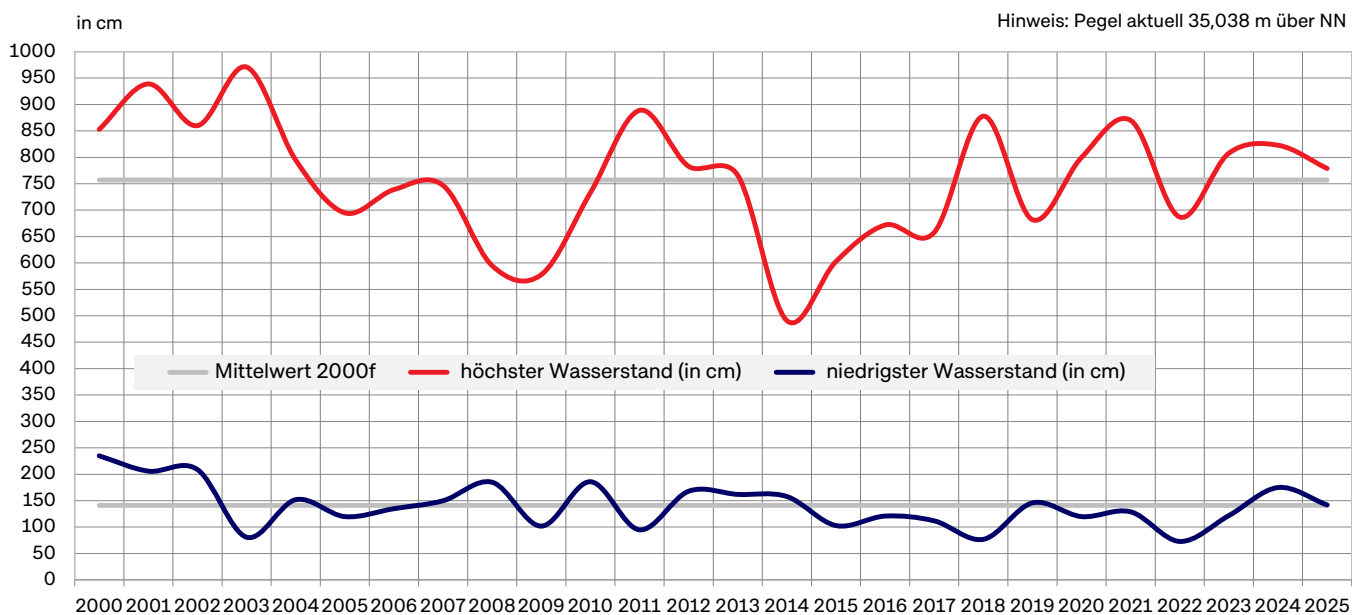
Grafik 003: Wasserstände des Rheins am Kölner Pegel (Rheinkilometer 688)
