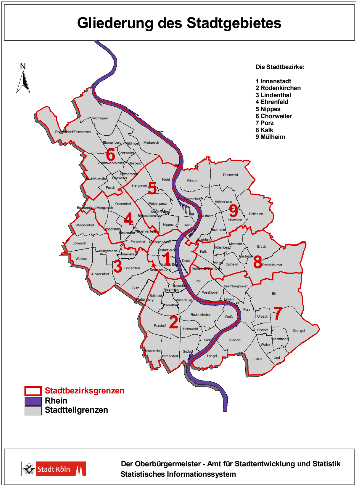
Karte 1002: Stadtgebiet Köln
