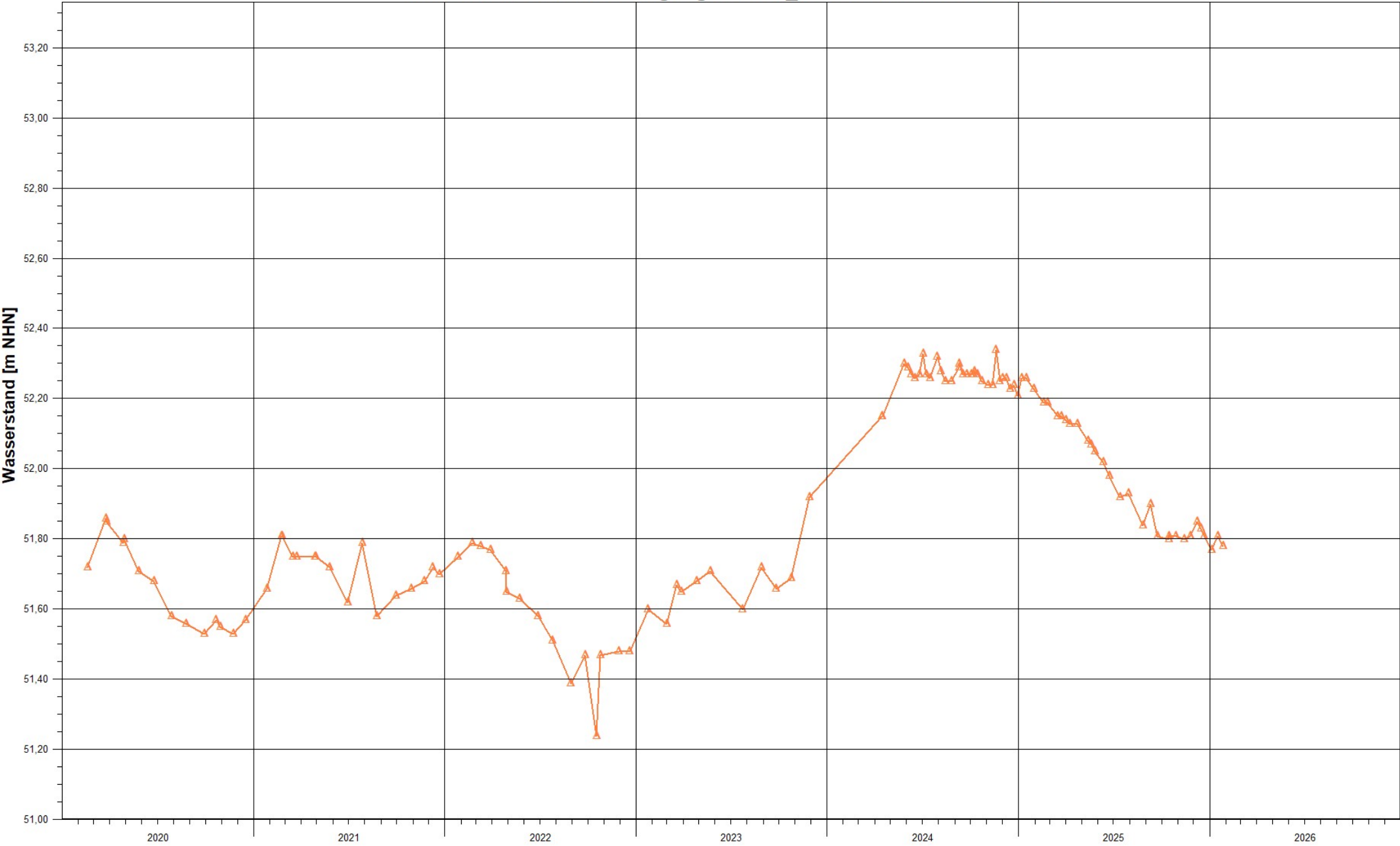
076748315, Grundwasserganglinie RS_47 01.01.2020 - 27.01.2026
