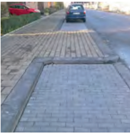
H1.1.6 Parkplatz - Standard
