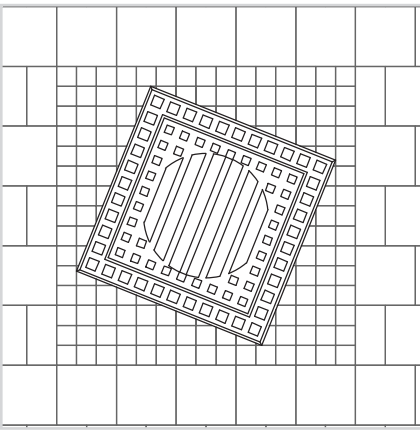
H1.3.2 Anordnung und Einbau (technischen) Elementen im Gehwegpflasterbelag - Standard für N
